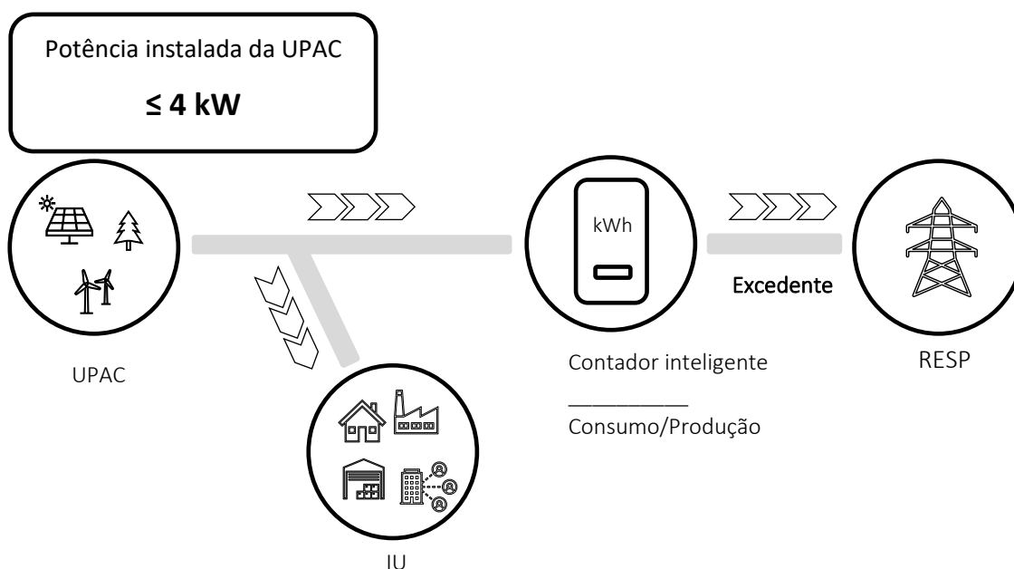
Figura 16 – UPAC de potência instalada, ≤ 4kW
